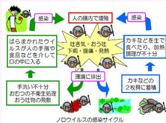
ノロウイルスの感染サイクル
